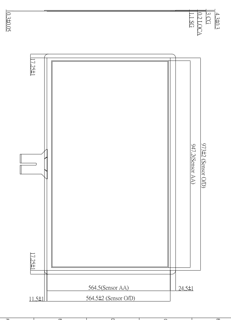
侧视图
