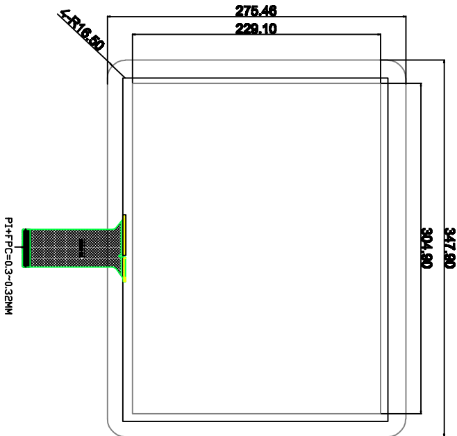
正视图
