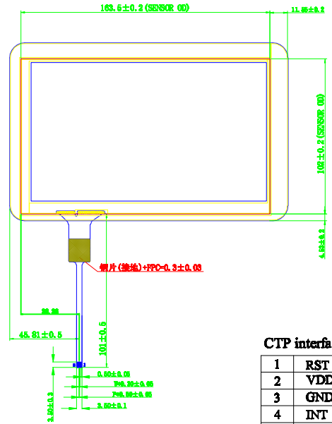
背面视图
