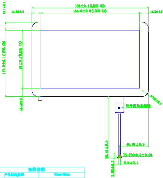
正面视图
