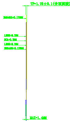
侧面视图
