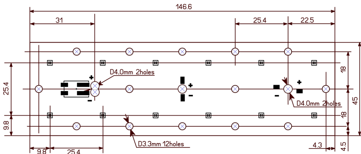
Рис. 2 Габаритные размеры светодиодного модуля ALC146.45.12-х-LH181B-XXXX-XX-05
