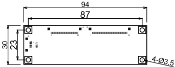
CONTROLLER SC 2:1
