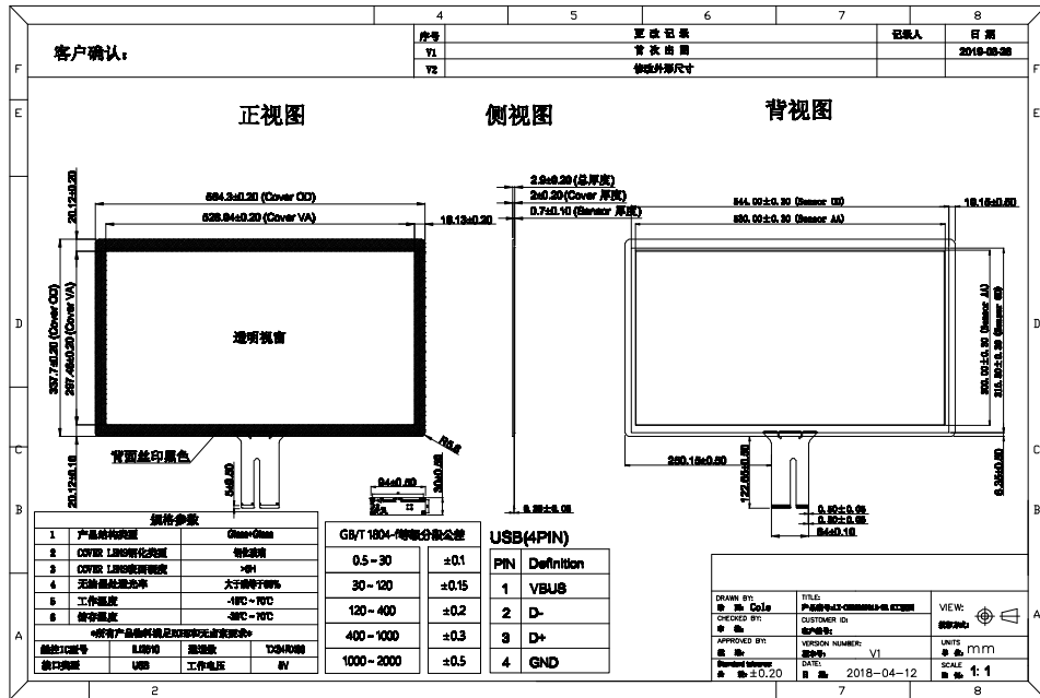
TP图纸:
