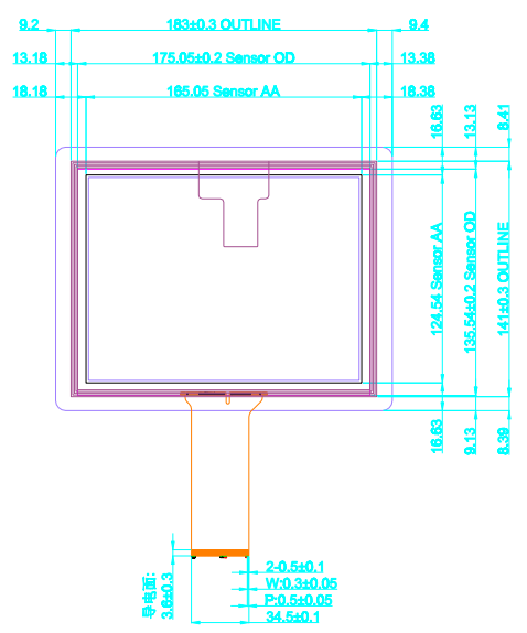
背视图
