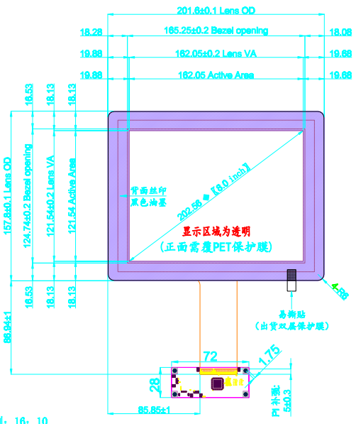
正视图
