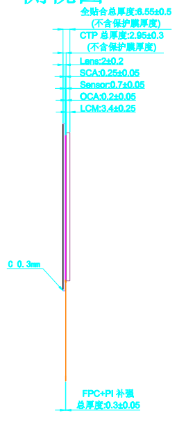
侧视图
