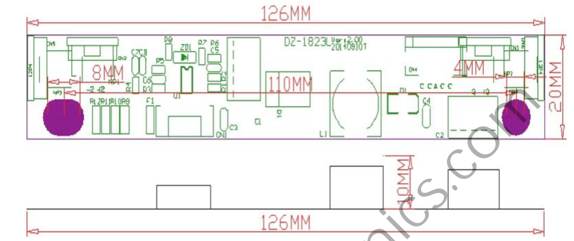
图 1-1 PCB 恒流板机械尺寸
