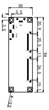
CONTROLLER SC 2:1
