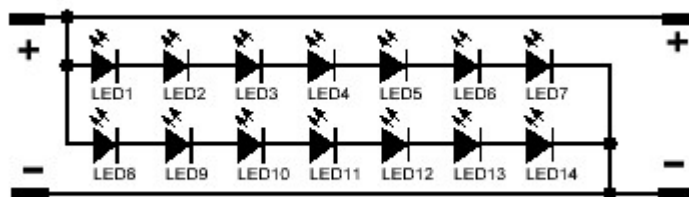
Рис. 1 Принципиальная схема светодиодного модуля ALS470.10-14-х-LM281Bp-XXXX-10
