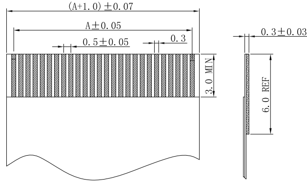
适用FPC寸法 APPLICABLE FPC
