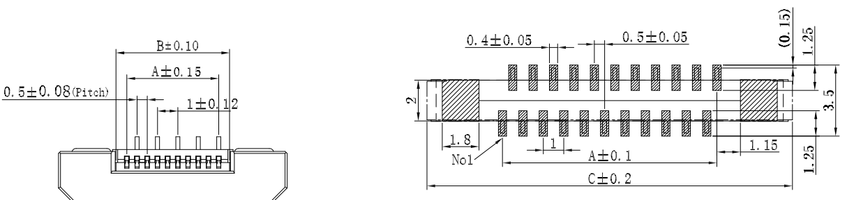
适用线路板 RECOMMENDED PCB LAYOUT
