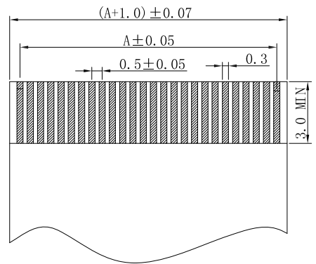
适用FPC寸法 APPLICABLE FPC
