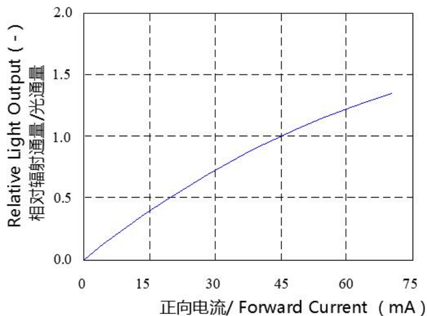
Forward Current vs. Light Output (Ta=25°C) 正向电流与辐射通量/光通量曲线图
