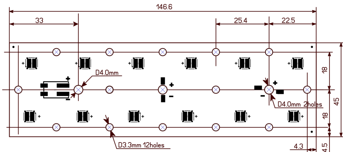
Рис. 2 Габаритные размеры светодиодного модуля ALC146.45.12-х-LH502C-XXXX-S 11 05
