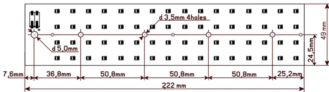
Рис. 2 Габаритные размеры светодиодного модуля ALC222.49.64-х-LM302D-XXXX
