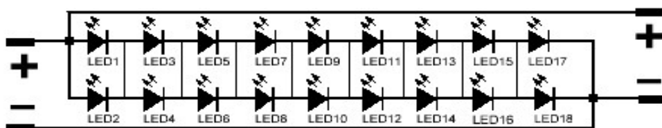
Рис. 1 Принципиальная схема светодиодного модуля ALS460.10-18-х-LM281Bp-XXXX-11
