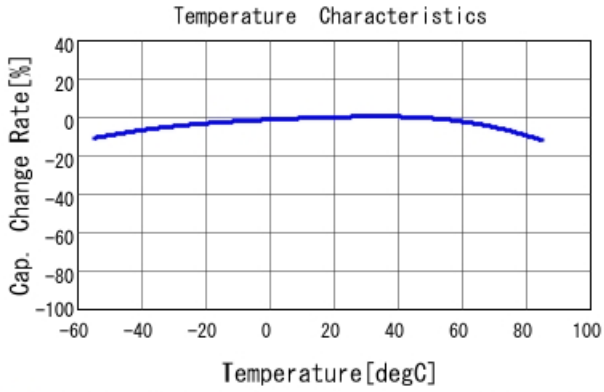
■ GRM31CR60J107MEA8 C-Temp. capchange, DCO. 0V, ACO. 2Vrm
