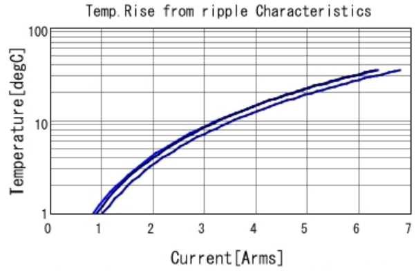
GRM31CR60J107MEA8 Temp. rise ■ 50kHz ■ 200kHz ■ 400kHz
