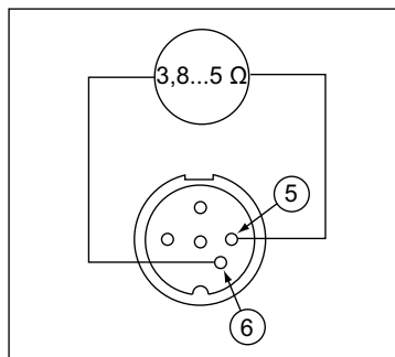
Штекер i-TOOL
