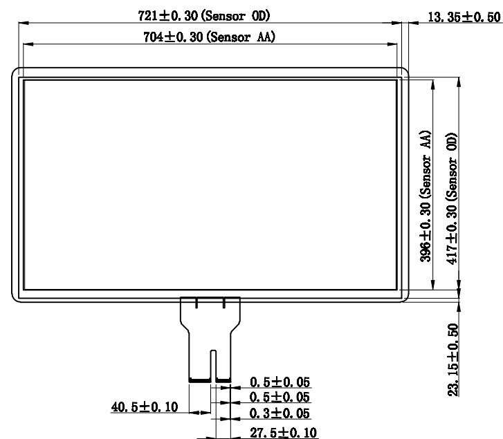
背视图
