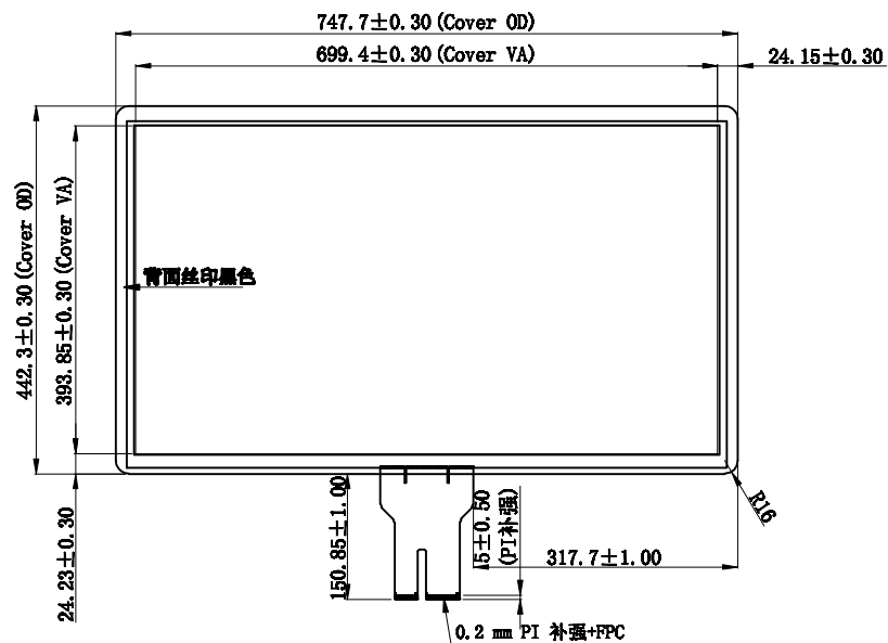
正视图
