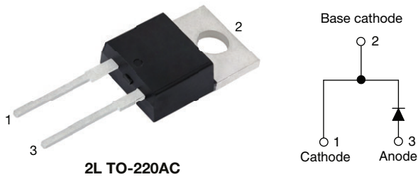
2L TO-220AC
