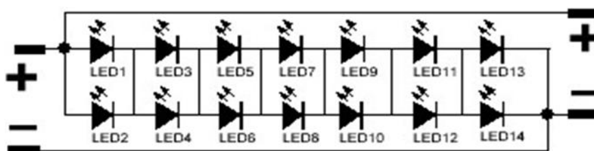
Рис. 1 Принципиальная схема светодиодного модуля ALS460.10-14-х-LM281Bp-XXXX-11
