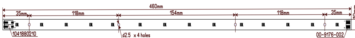
Рис. 2 Геометрические размеры светодиодного модуля ALS460.10-14-х-LM281Bp-XXXX-11
