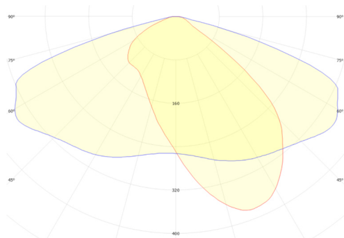
Клевер CLP-5050F5A FWHM = 146°×61°, \eta = 94,4 %
