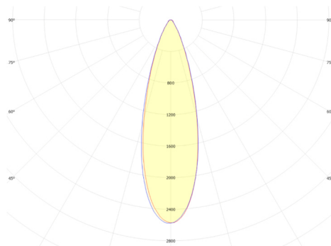
GSLED 5050.V6X.40 FWHM = 30°, \eta = 91,9 %
