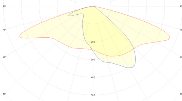
GSLED 5050.V6X.40 FWHM = 148°×60°, \eta = 97,9 %
