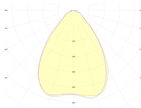
GSLED 5050.V6X.20 FWHM = 77°, \eta = 95,1 %
