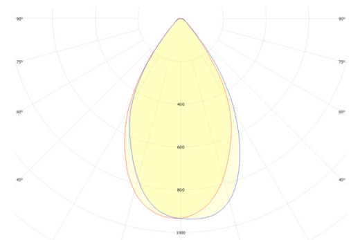
OSRAM DURIS S8 FWHM = 60°, \eta = 94,1 %
