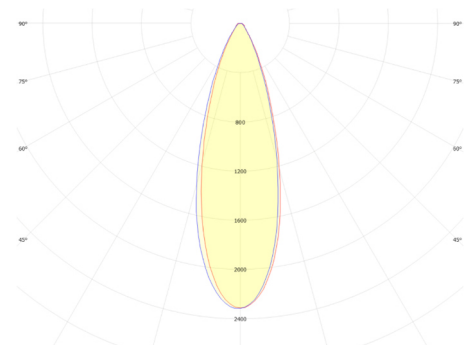
OSRAM DURIS S8 FWHM = 31°, \eta = 90,7 %
