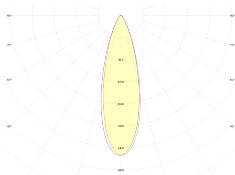
Клевер CLP-5050F5A FWHM = 30°, \eta = 92,1 %
