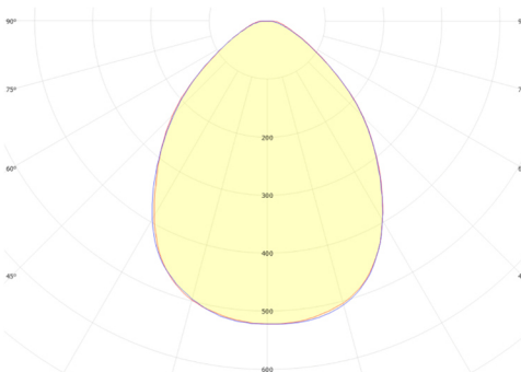
Seoul STW0L8PA FWHM = 84°, \eta = 92,2 %
