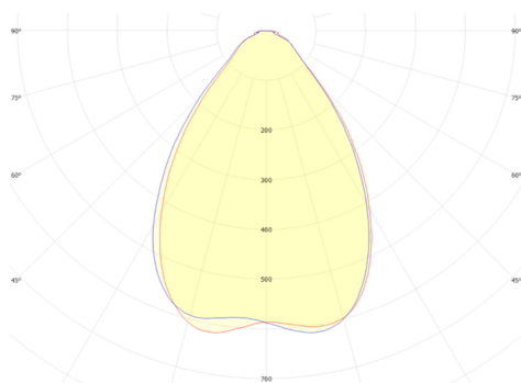
Клевер CLP-5050F5A FWHM = 73°, \eta = 94,7 %
