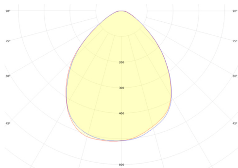
GSLED 5050.V6X.40 FWHM = 87°, \eta = 92,6 %
