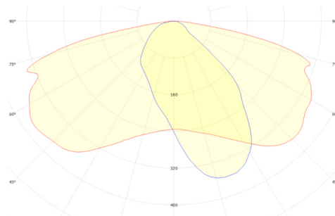
OSRAM DURIS S8 FWHM = 157°×59°, \eta = 95,7 %
