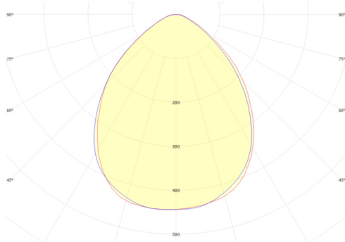
GSLED 5050.V6B.50 FWHM = 90°, \eta = 90,2 %
