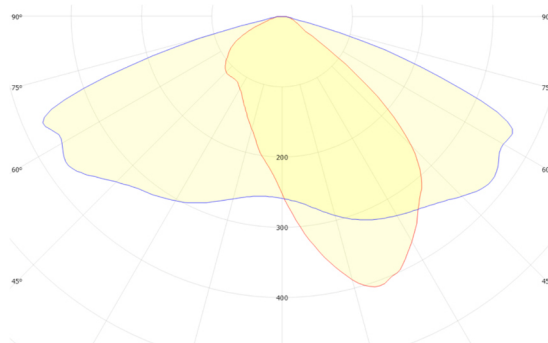
OSRAM DURIS S8 FWHM = 144°×56°, \eta = 92,8 %
