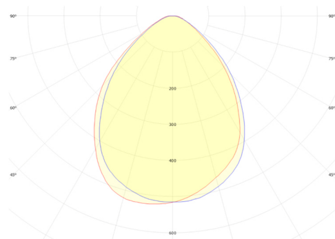
GSLED 5050.V6X.41 FWHM = 86°, \eta = 91,5 %
