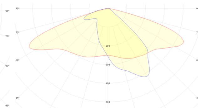
OSRAM DURIS S8 FWHM = 146°×55°, \eta = 97,3 %
