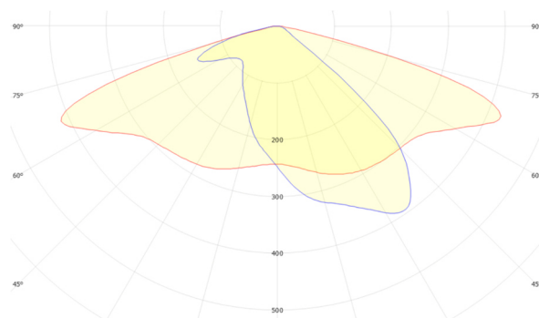
Клевер CLP-5050F5A FWHM = 148°×61°, \eta = 98,8 %
