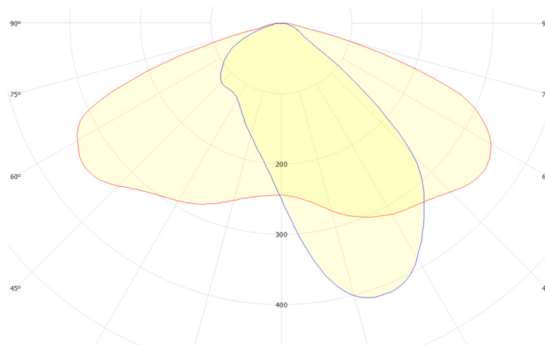
OSRAM DURIS S8 FWHM = 143°×54°, \eta = 95,5 %
