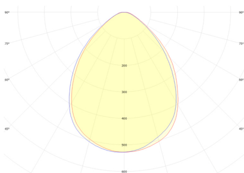
Клевер CLP-5050F5A FWHM = 85°, \eta = 93,2 %
