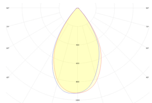
GSLED 5050.V6B.50 FWHM = 61°, \eta = 91,9 %
