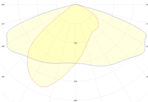
GSLED 5050.V6X.40 FWHM = 146°×64°, \eta = 93,3 %
