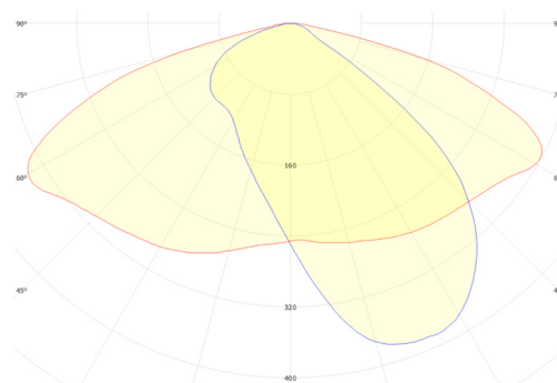
GSLED 5050.V6X.20 FWHM = 148°×61°, \eta = 95,2 %
