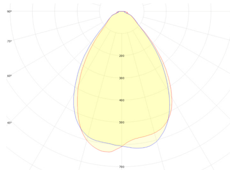
GSLED 5050.V6X.41 FWHM = 71°, \eta = 94,3 %
