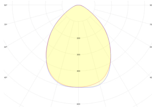
OSRAM DURIS S8 FWHM = 87°, \eta = 92,1 %
