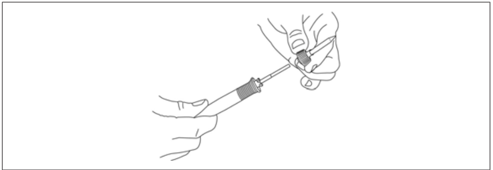
图 2: 取下焊头
