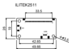
CONTROLLER SC 2:1
