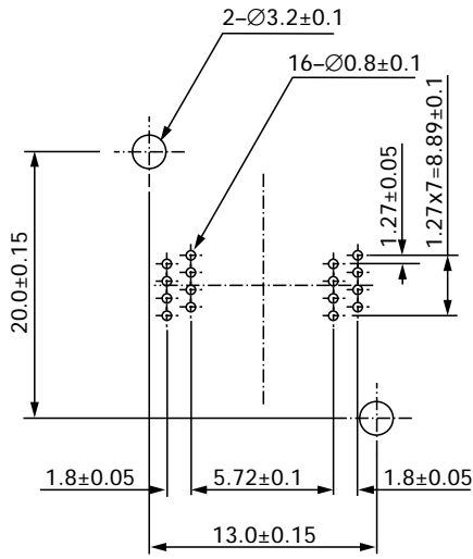
16 pins (SOP) IC51-0162-273-1
