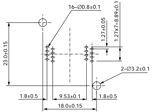
16 pins (SOP) IC51-347.KS-7704
