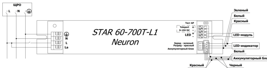
Рисунок 9 – Схема подключения БАП
