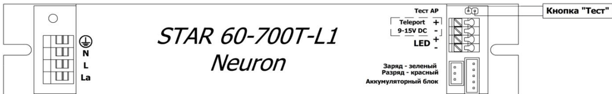
Рисунок 10 – Схема подключения кнопки «Тест»
