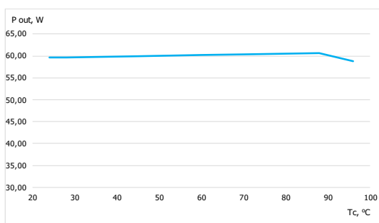
Рисунок 6 – Зависимость выходной мощности в рабочем режиме от T_c °C корпуса в точке T_c (при U_{in} = 230 VAC)
