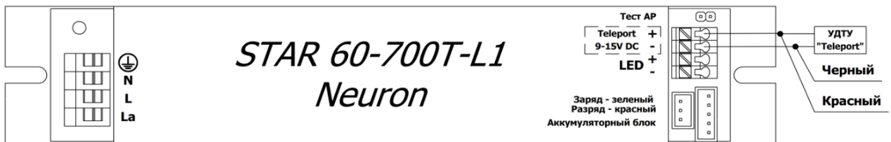
Рисунок 11 – Схема подключения УДТУ «Teleport»
