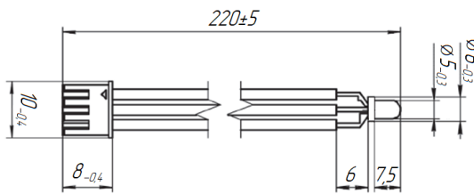
в) LED-индикатор
