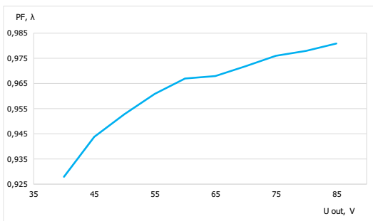
Рисунок 2 – Зависимость коэффициента мощности от выходного напряжения (при U_{in} = 230 \text{ VAC} )
