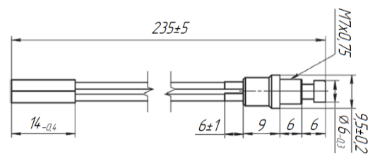
г) Кнопка «Тест»
