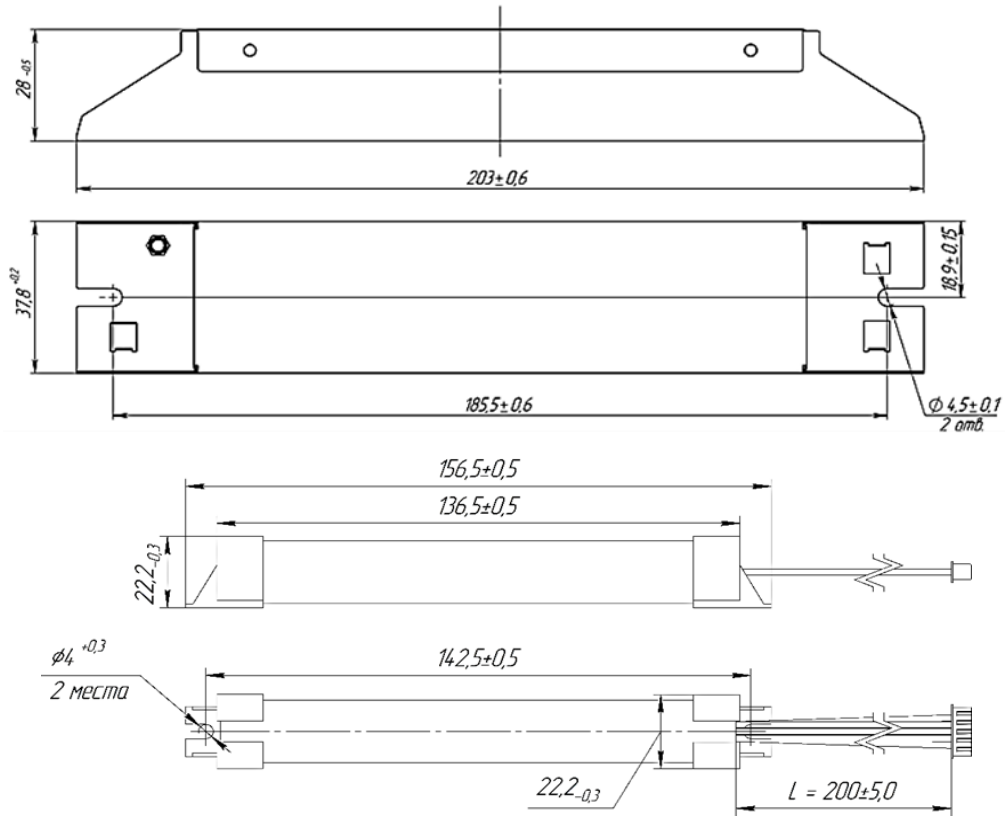
а) Блок аварийного питания и аккумуляторный блок
