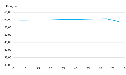
Рисунок 5 – Зависимость выходной мощности в рабочем режиме от T_c °C окружающей среды (при U_{in} = 230 VAC)
