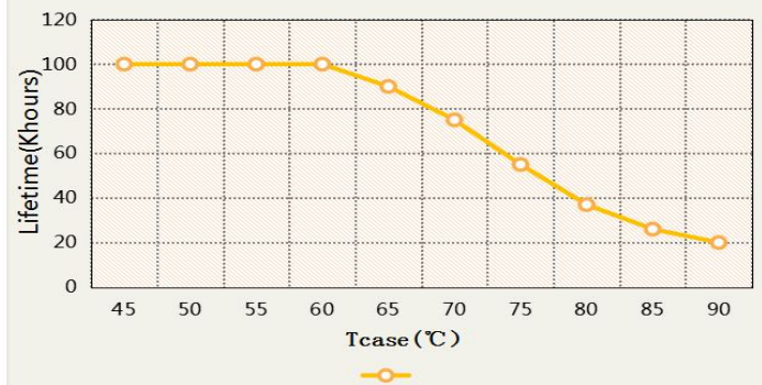
Tcase VS Lifetime 壳温 VS 寿命
